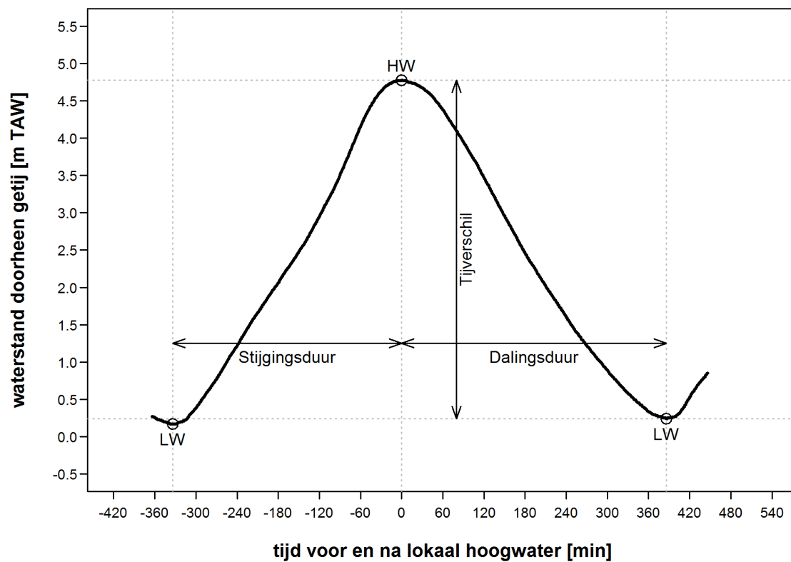
Figuur 7: Aanduiding van getijkenmerken op een getijkromme
