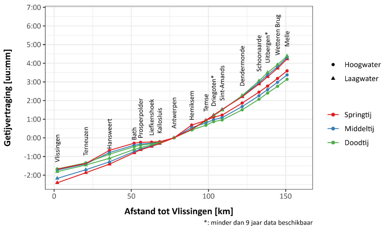
Figuur 15: Getijvertraging HW en LW langs de Westerschelde en Zeeschelde over het decennium 2011-2020 bij middeltij, springtij en doodtij
