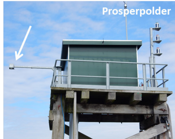
Figuur 2: Opstelling radar voor de getijposten Antwerpen (links) en Prosperpolder (rechts)
